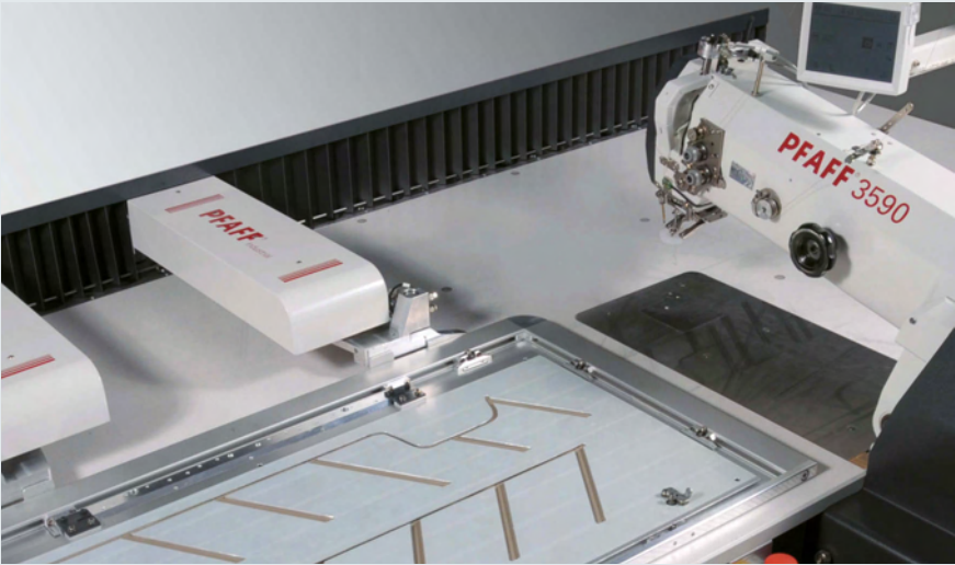
Parallelnähte für Tür-Innenverkleidungen
